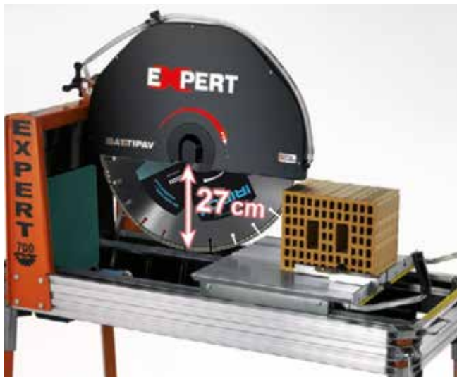
CORTES EN RECTO Posición de corte con carro deslizante. (Expert 9700).
