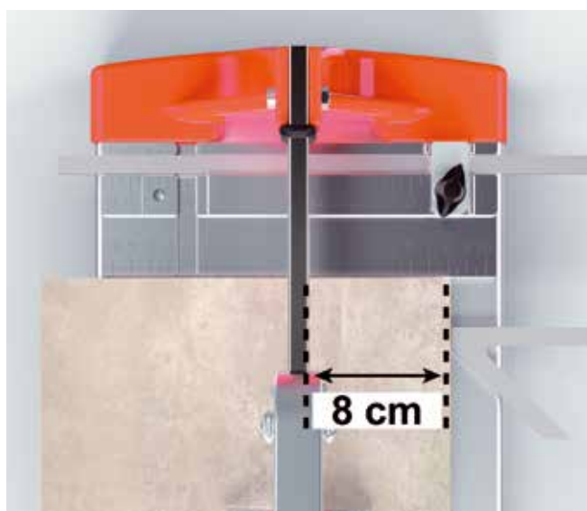
CORTE RECTO Regla cuadrada con lectura directa para cortes rectos.
